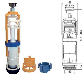
VÁLVULA DESCARGA OLI POUSSOIR C/ADAPT. ROCA
