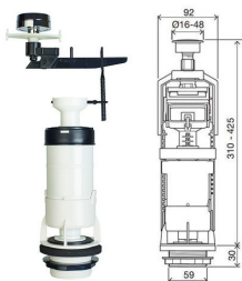
VÁLVULA DESCARGA OLI POUSSOIR ECO
